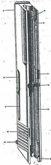
Obr. 6. Závěr 1 - muška, 2 - hledí, 3 výhozne okénko, 4 - vybrání pro vytahovač, 5 - lůžko pro hlaveň, 6 - lišty, 7 - vybrání pro ozub záchytky závěru, 8 - vybrání pro uzamykací váleček, 9 - vybrání pro přerušovač
