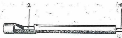
Obr. 7. Úderník 1 - zápalkník, 2 - vybrání pro pojistku úderníku
