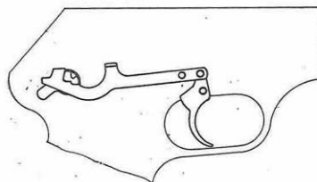
Obr. 44. Poloha součástí odjištěné pistole
