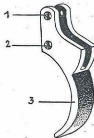
Obr. 23. Spoušť 1 - otvor pro kolík přerušovače, 2 - otvor pro kolík spouště, 3 - jazýček
