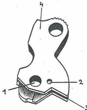
Obr. 26. Kohoutek 1 - otvor pro čep kohoutku, 2 - otvor pro kolík kohoutku, 3 - výřez pro údernou zpruhu a její vodičí tyčinku, 4 - hlava kohoutku
