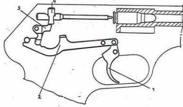
Obr. 45. Poloha součástí při zajištěném úderníku 1 - spoušť, 2 - přerušovač, 3 - spoušťová páka, 4 - pojistka úderníku
