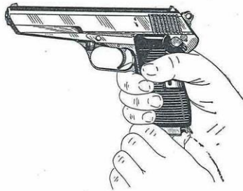
Obr. 50. Vyjímání zásobníku z pistole
