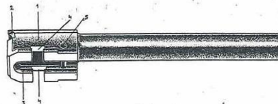
Obr. 2. Hlaveň
