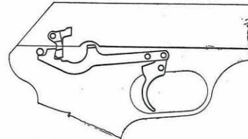
Obr. 48. Poloha přerušovače před výstřelem
