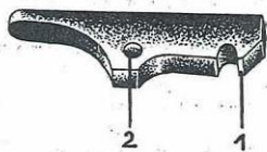
Obr. 10. Vytahovač 1 - drápek vytahovače, 2 - otvor pro kolík vytahovače
