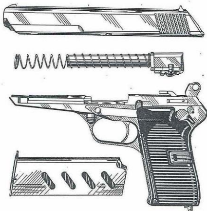
Obr. 53. Neúplně rozebraná pistole
