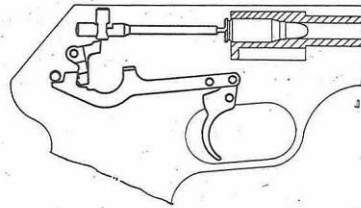
Obr. 46. Poloha součástí při odjistěném úderníku
