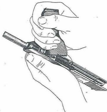
Obr. 54. Zasunutí hlavně do závěru
