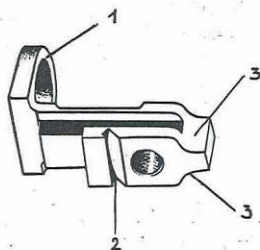
Obr. 3. Uzamykač 1 - kruhová objímka, 2 - příčný zářez, 3 - čtverhrubé vybrání pro uzamykač
